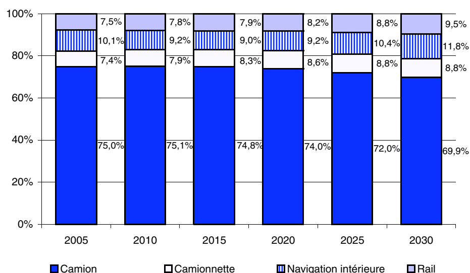
GRAPHIQUE 31 - Parts des moyens de transport dans le nombre de tonnes-kilomètres – transport national de marchandises – scénario de référence
