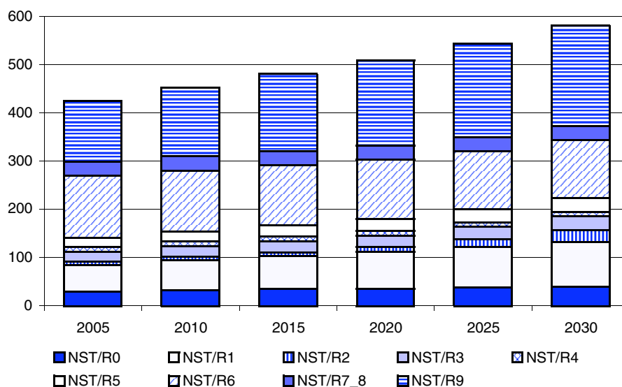
GRAPHIQUE 23 - Tonnage transporté – Transport national de marchandises (millions de tonnes) – scénario de référence
