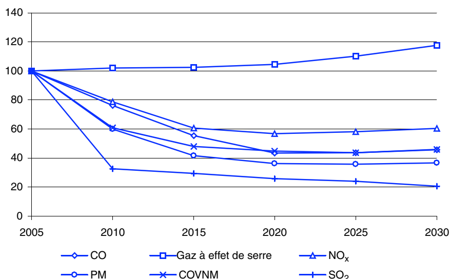
GRAPHIQUE 34 - Emissions directes du transport de personnes et de marchandises en Belgique (route, rail, navigation intérieure) – 2005=100 – scénario de référence
